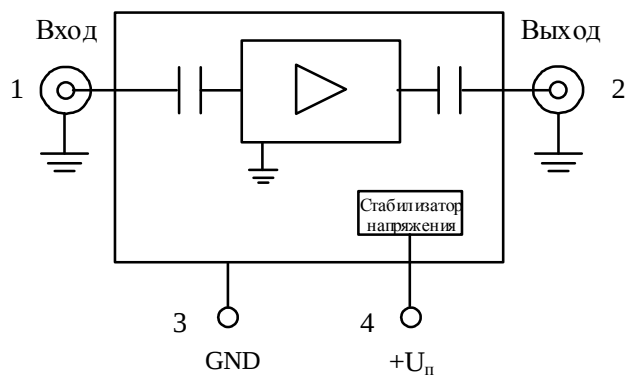
Функциональная схема усилителя МАНВ-010120
