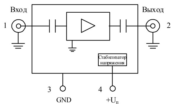
Функциональная схема усилителя МАНВ-040100
