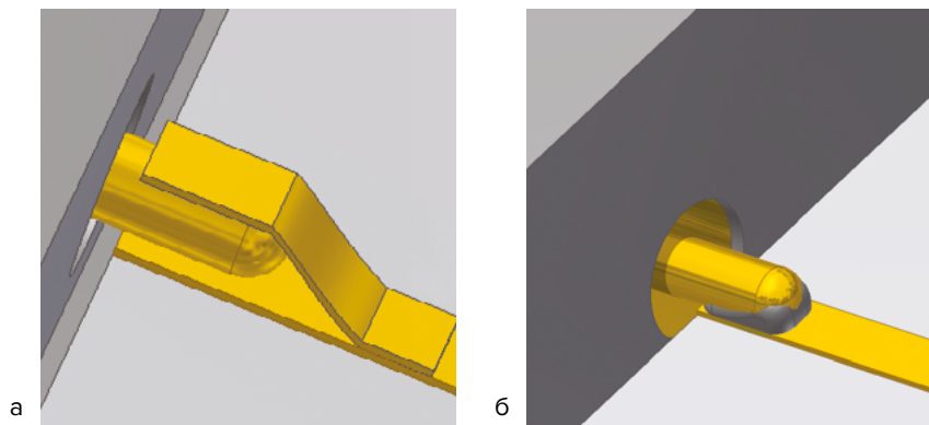
Рис. 51. Способы соединения гермоввода с микрополосковой линией
