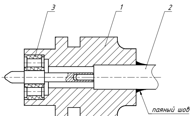
Рис. 25. Запрессовка диэлектрической опоры в кабельный соединитель
