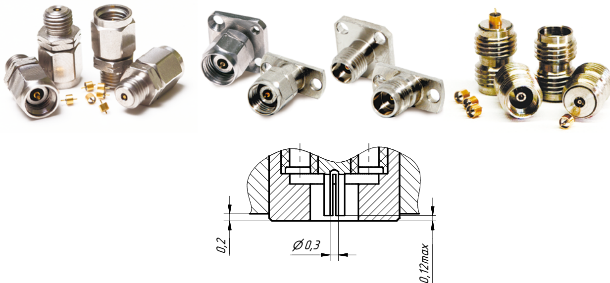
Рис. 8. Вид гнезда с приборной стороны КМПП
