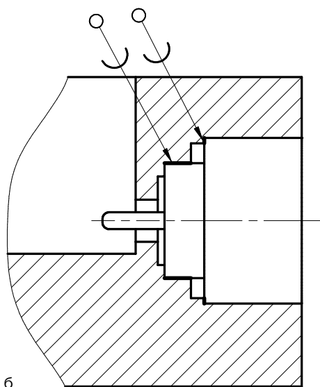
Рис. 21. Рекомендуемое установочное отверстие (а) и установка (б) КМПП ПКМ2-26-16-0,38/1,27
