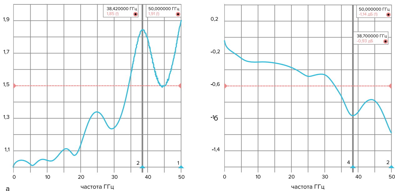
Рис. 49. Частотные характеристики экспериментальной сборки: КСВН (а) и коэффициент передачи (б)
