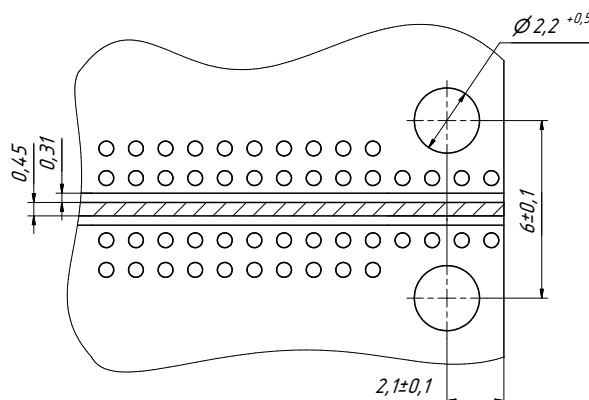
Рис. 17 – Топология платы
