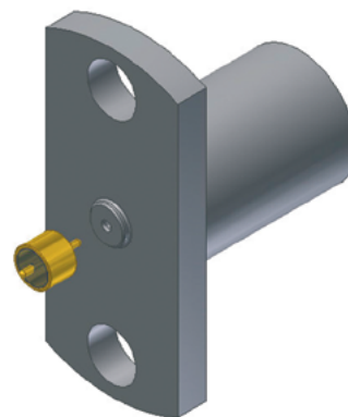
Рис. 7. Приспособление для пайки гермоввода для устройств, использующих фланцевый корпус КМПП с двумя крепежными отверстиями (ЖНКЮ.731424.001 Упор)
