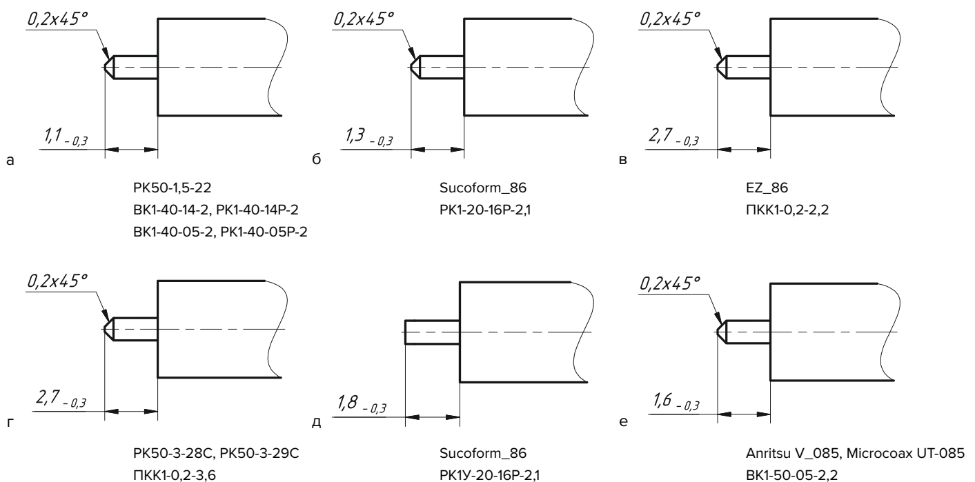
Рис. 22. Разделка кабеля
